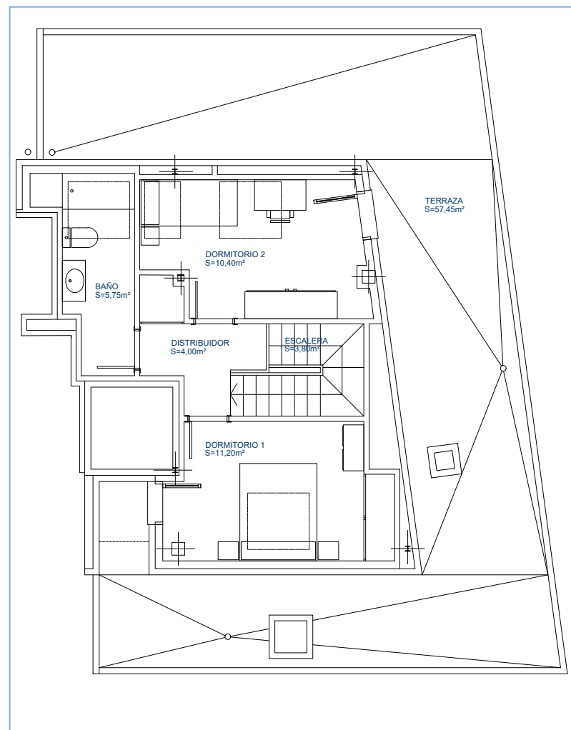
PLANTA SEGUNDA
